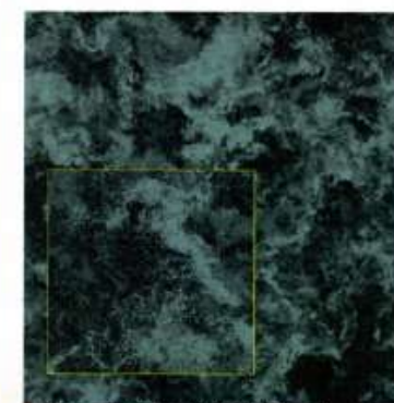
世界最大規模乱流直接数値シミュレーション (格子点数122883)により得られた高レイノルズ数乱流中の渦の組織構造 名古屋大学附属計算科学連携教育研究センター
