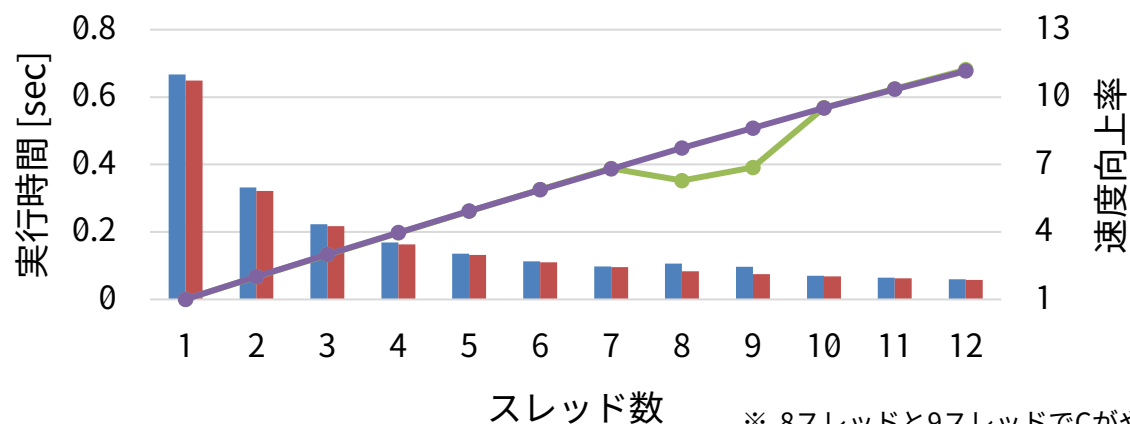
行列ベクトル積
