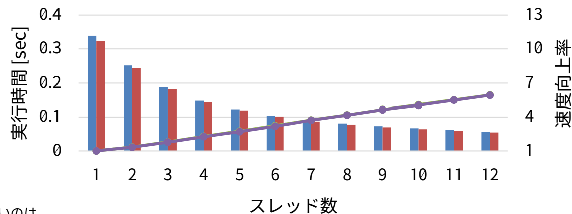
三角行列ベクトル積
