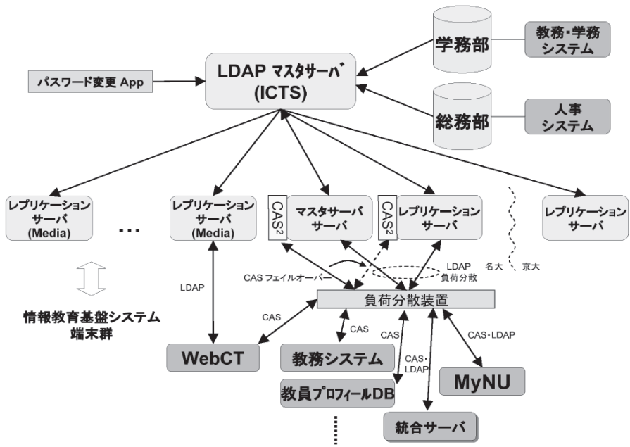
図3 名古屋大学 ID サーバの構成 (現在)
