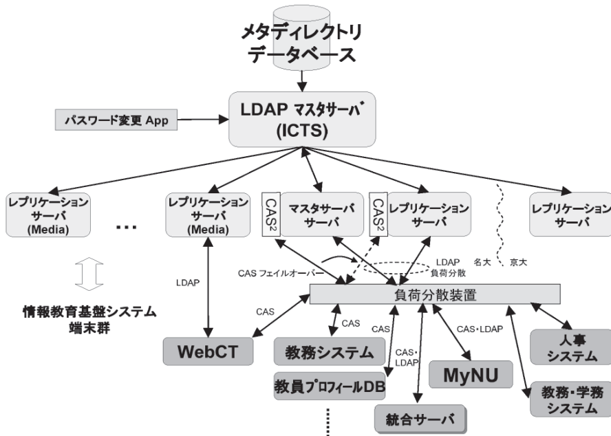
図4 名古屋大学 ID サーバの構成 (数年後)
