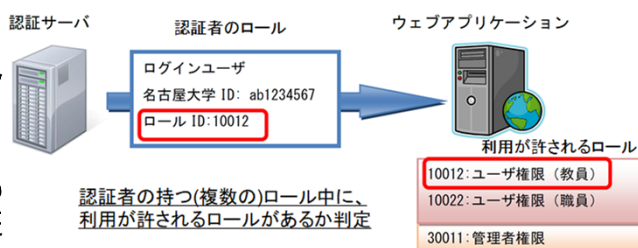
ロール情報も併用したシングルサインオン
